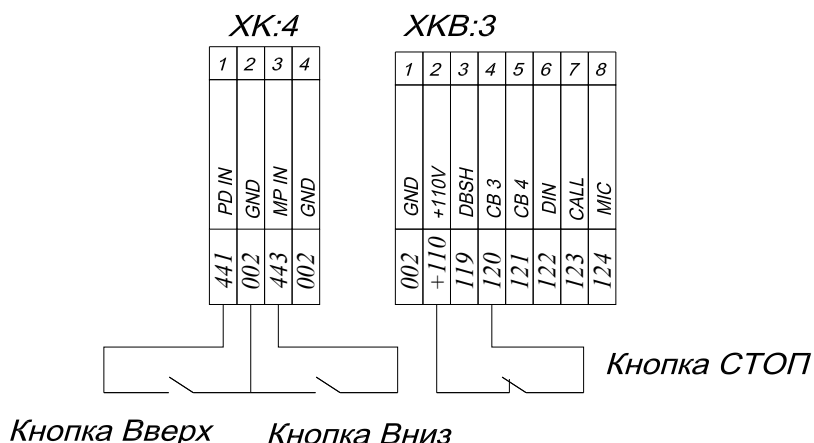
Рис. 2 Подключение поста ревизии.
