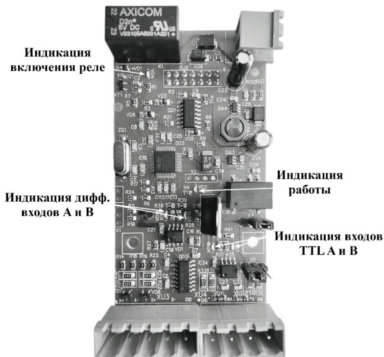
Рис. 7 Плата УКСЛ
