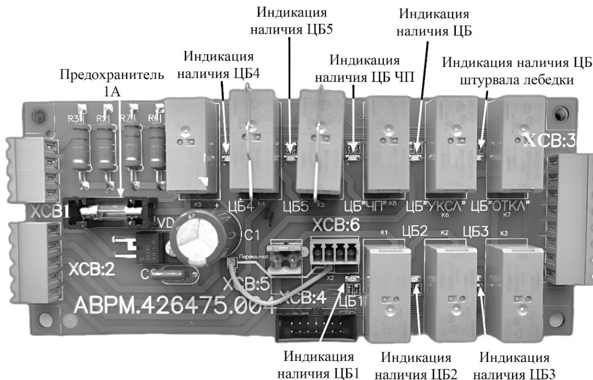
Рис. 5 Плата ЦБ
