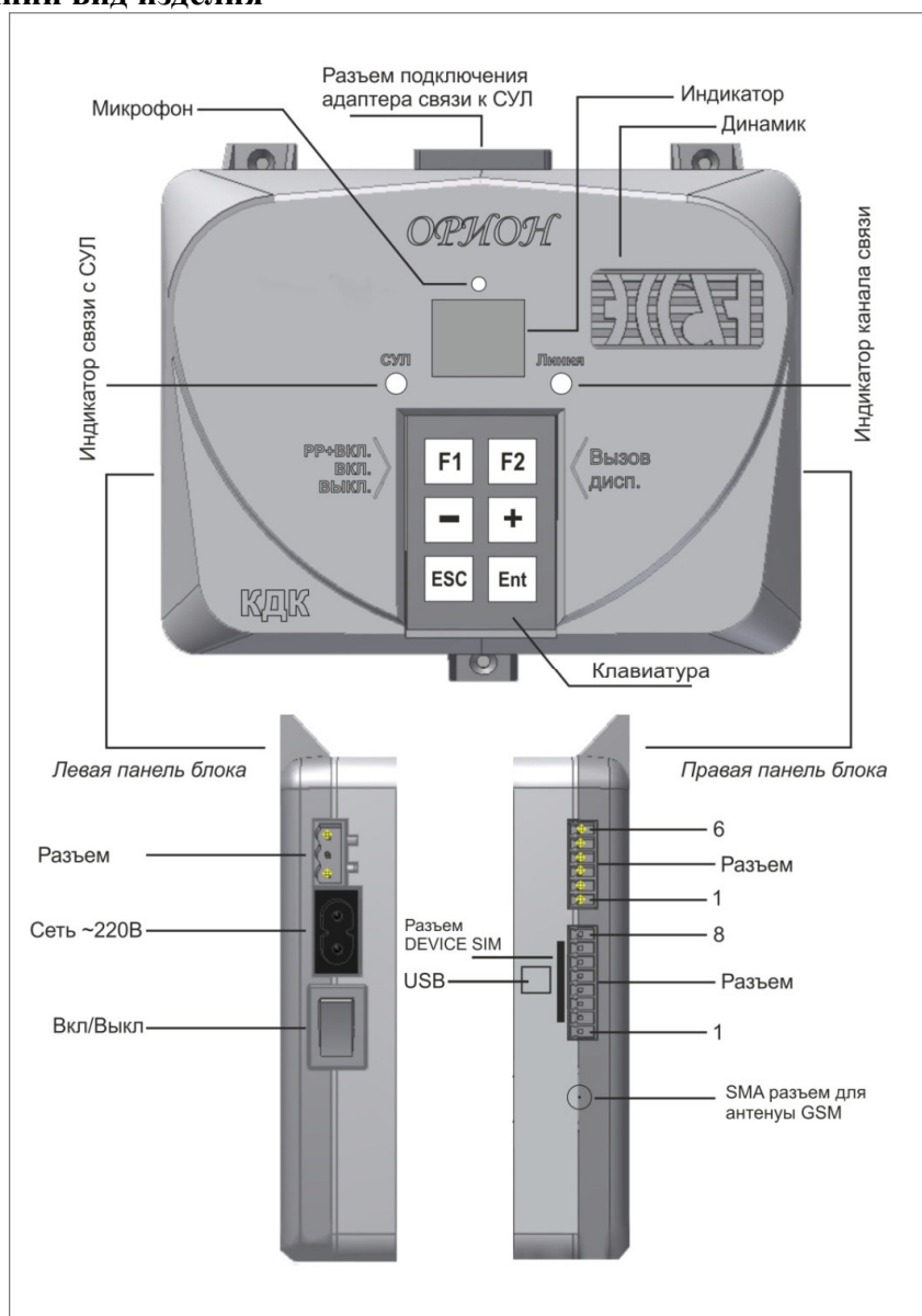
Рис. 1 Лифтовой Блок «Орион GSM»
