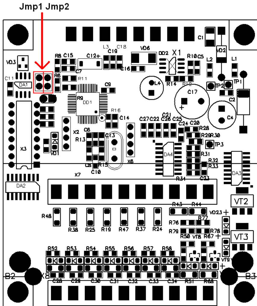
Рис. 29 Установка перемычек для подключения согласующих резисторов.
