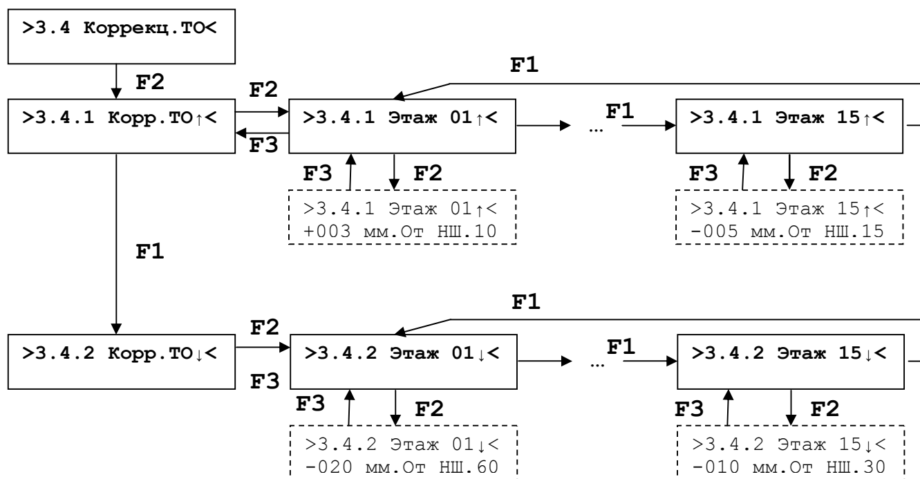
Рис. 25 Структура подменю >3.4 Коррекц.ТО<
