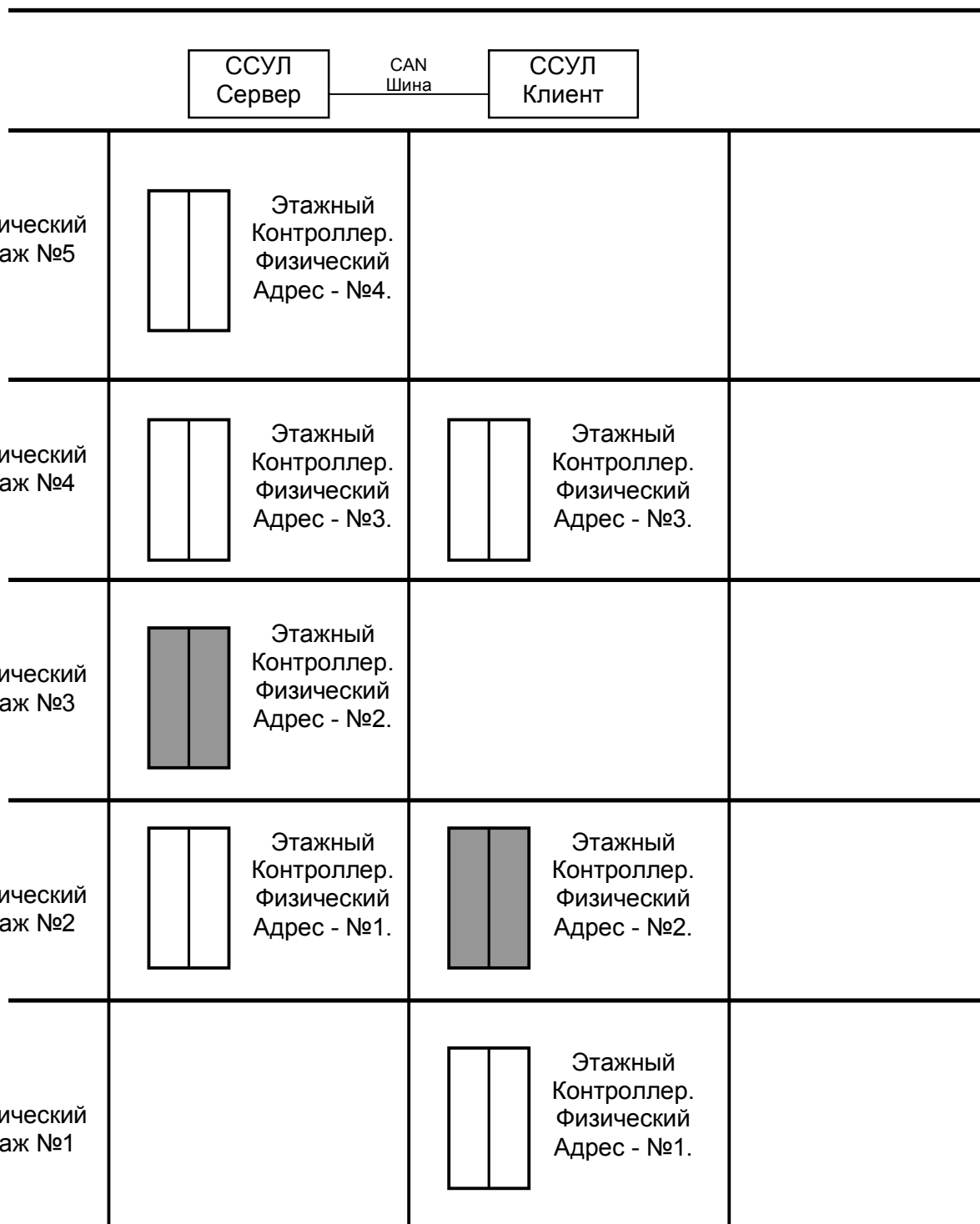
Рис. 32 Конфигурация №3. Задание адресов Этажных контроллеров и Логических Этажей.
