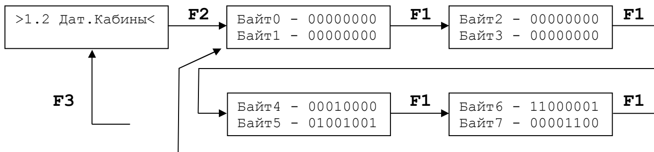
Рис. 9 Структура подменю >1.2 Дат. Кабины<
