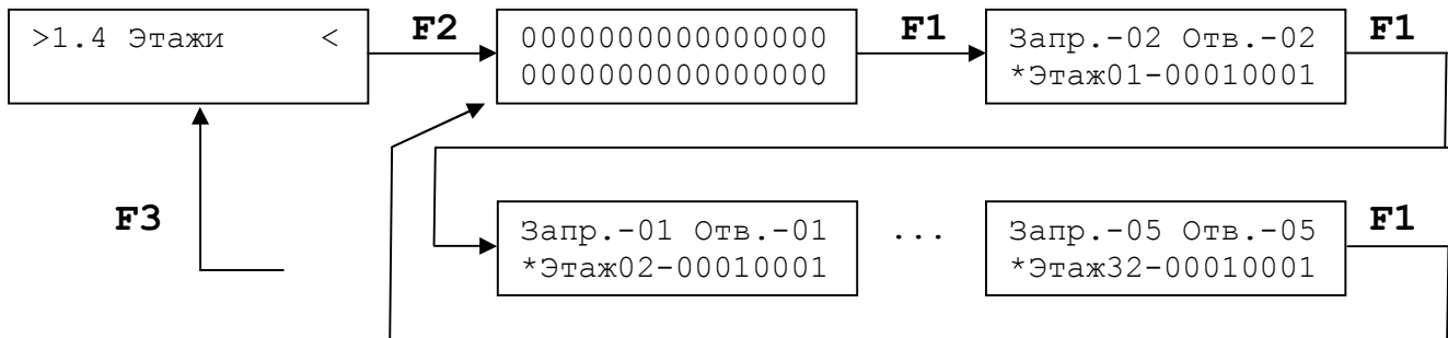
Рис. 10 Структура подменю >1.4 Этажи <
