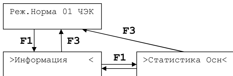
Рис. 5 Структура меню в режиме «НОРМА».
