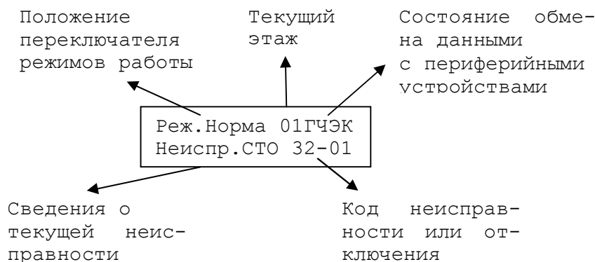
Рис. 4 Информация на индикаторе.
